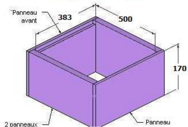
Corps de ruche DADANT 10c
