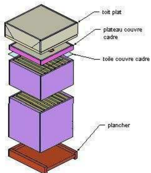
Ruche DADANT
