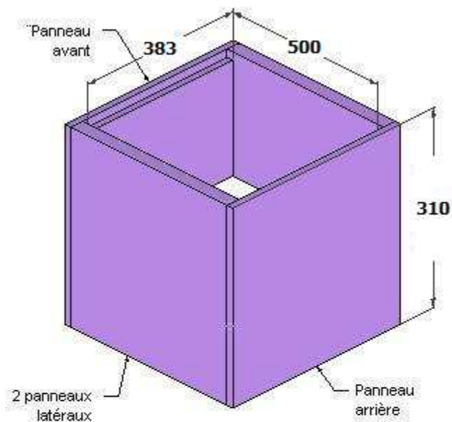
Corps de ruche DADANT 10c
